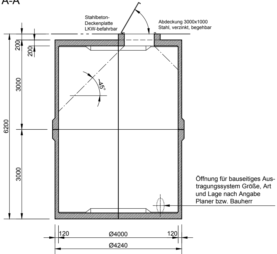
Schnitt A-A
