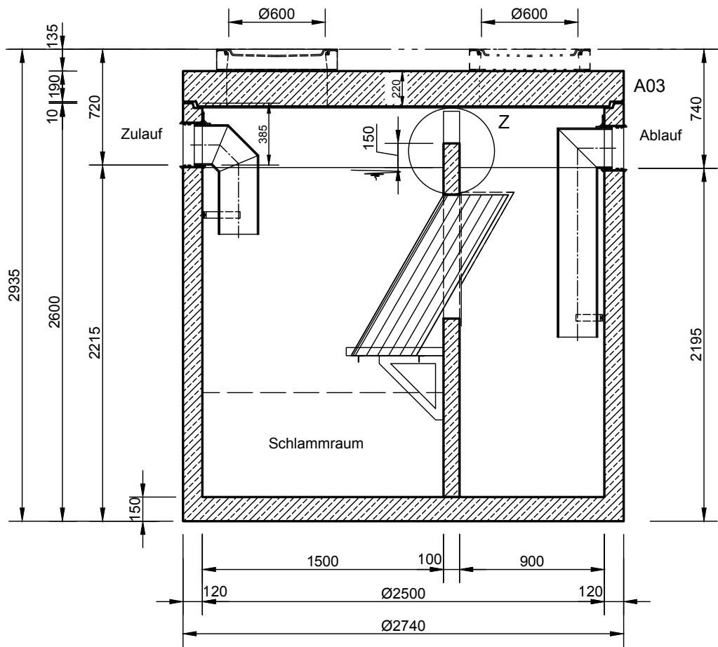
Schnitt A-A
